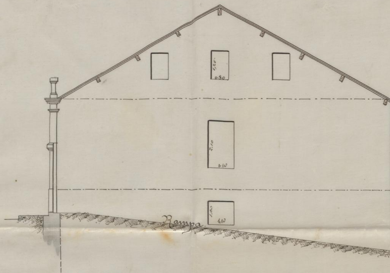
Alçado lateral
