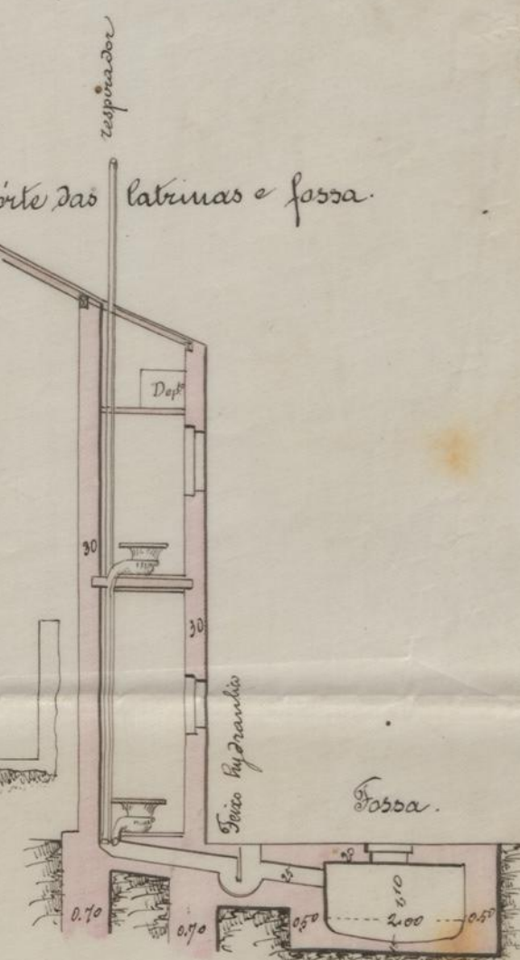
Corte da fossa.
