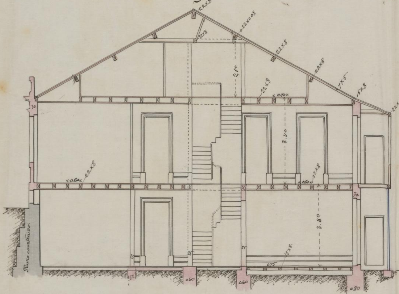
Corte longitudinal.
