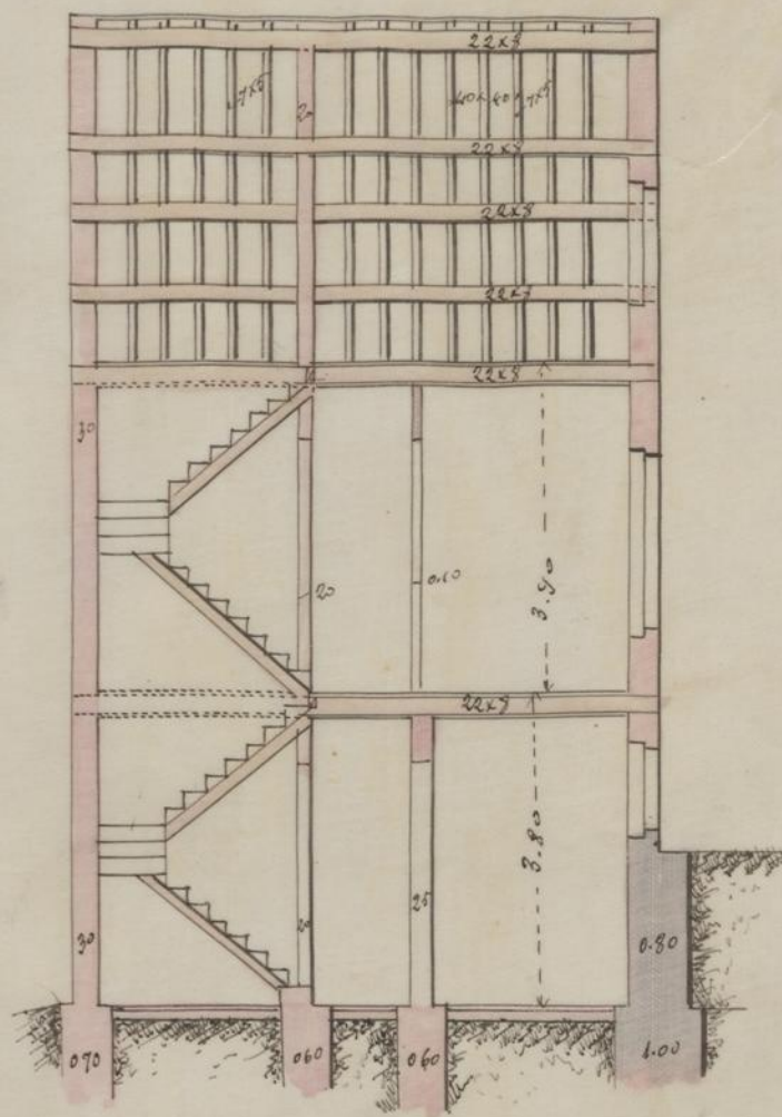
Corte transversal.
