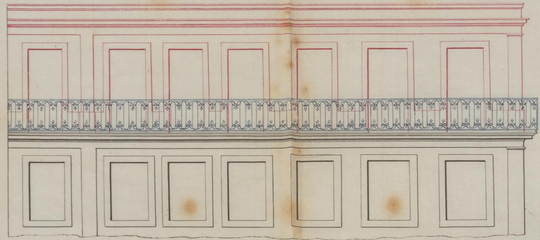
Alçado do lado do Sul, sobre o Passeio das Fontainhas
