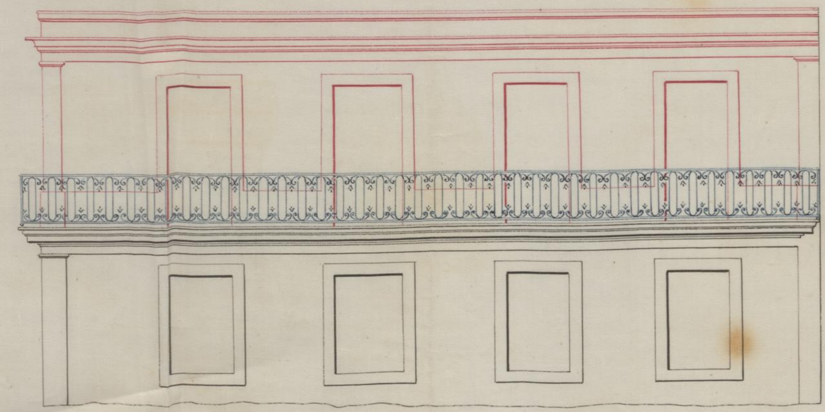
Alçado do lado do Nascente, sobre a rua das Fontainhas.
