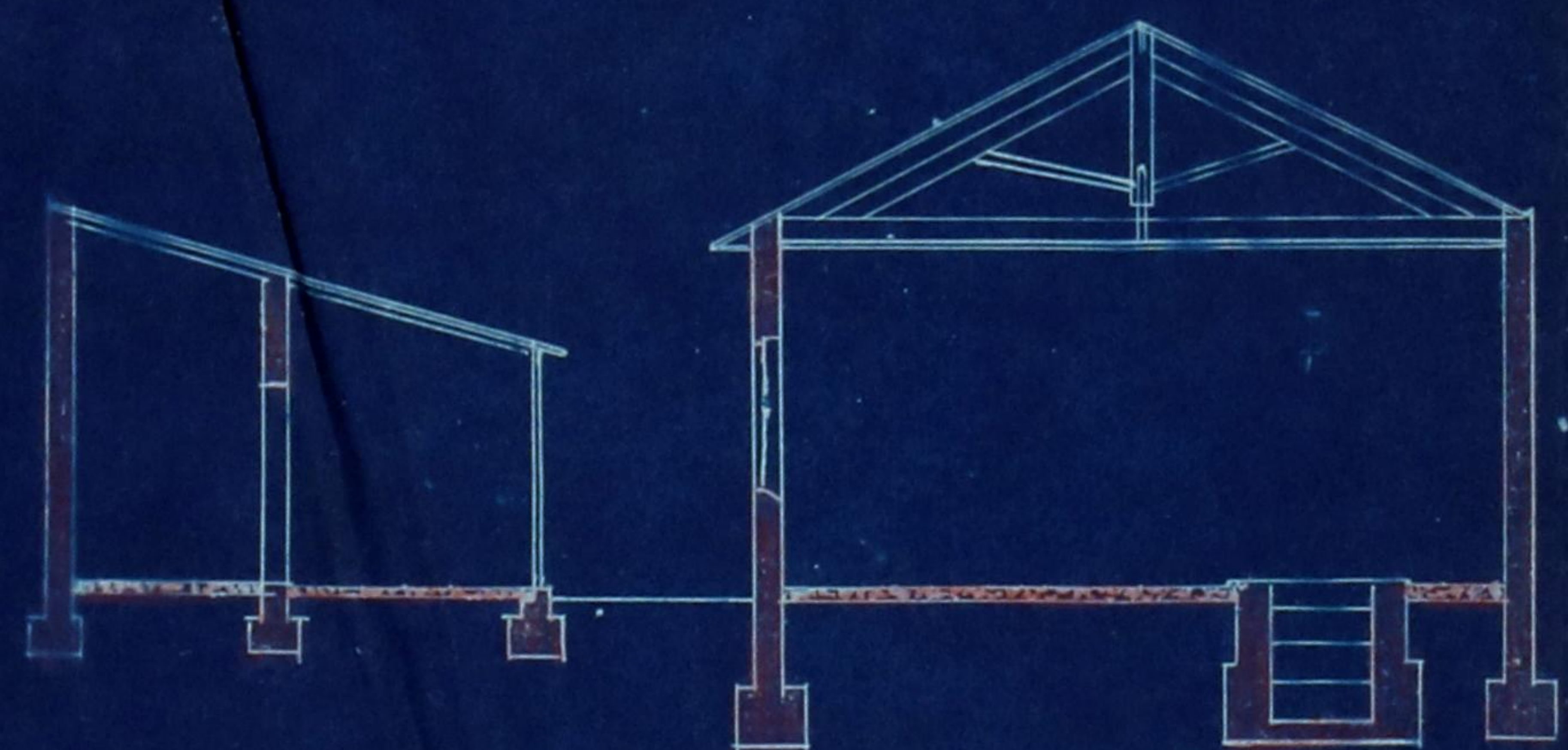
Secção transversal
