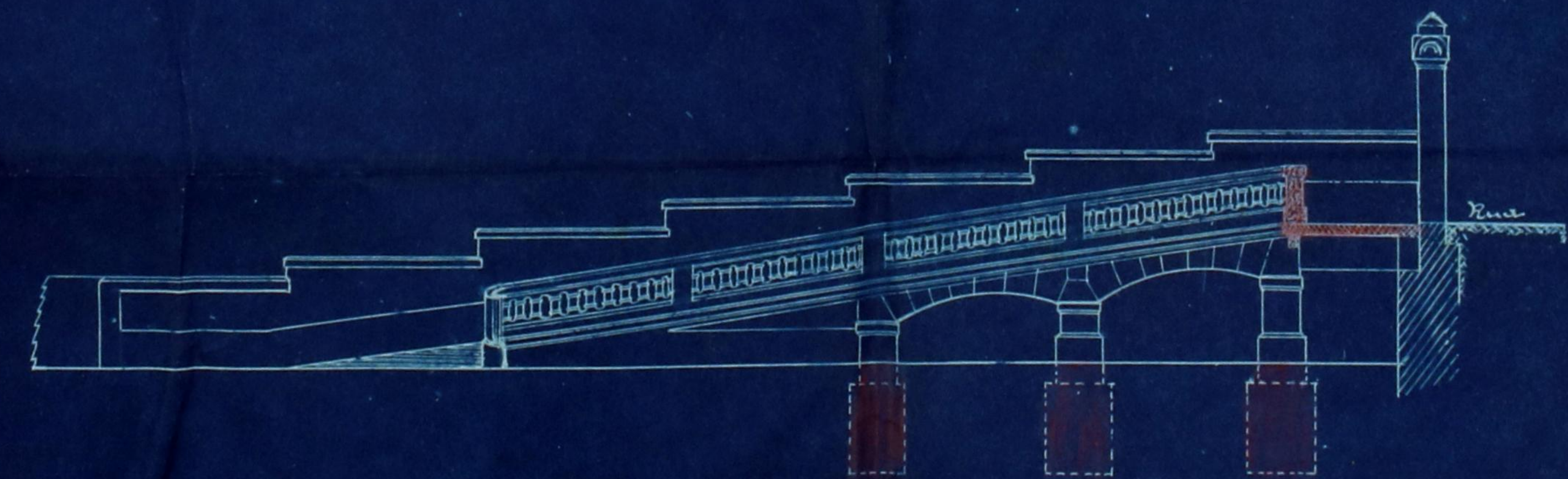
Fachada da rampa
