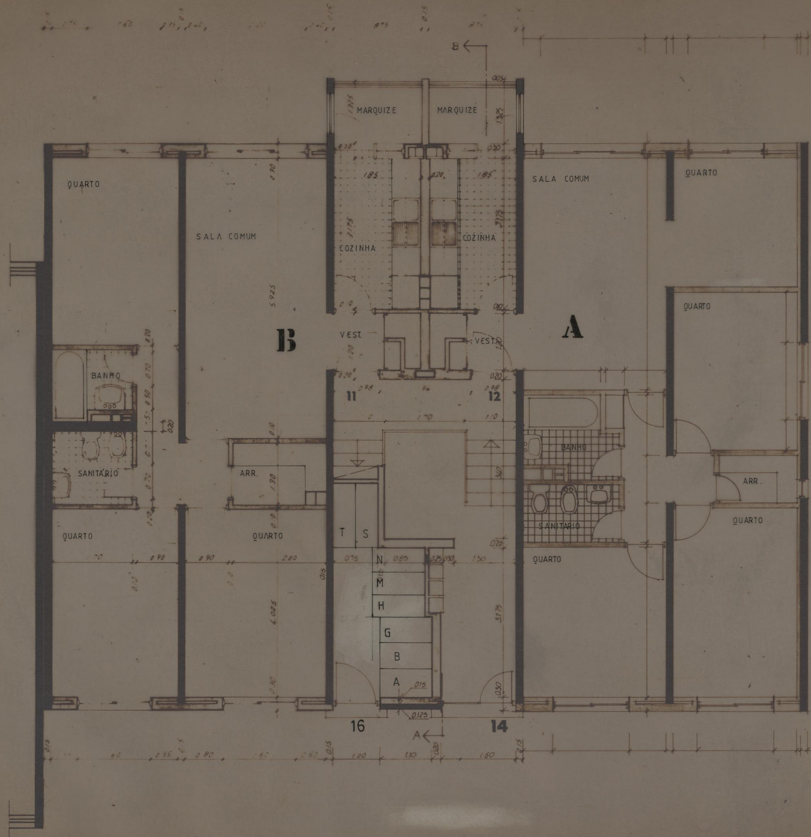
PLANTA DO R/CHÃO (edificio 2)
