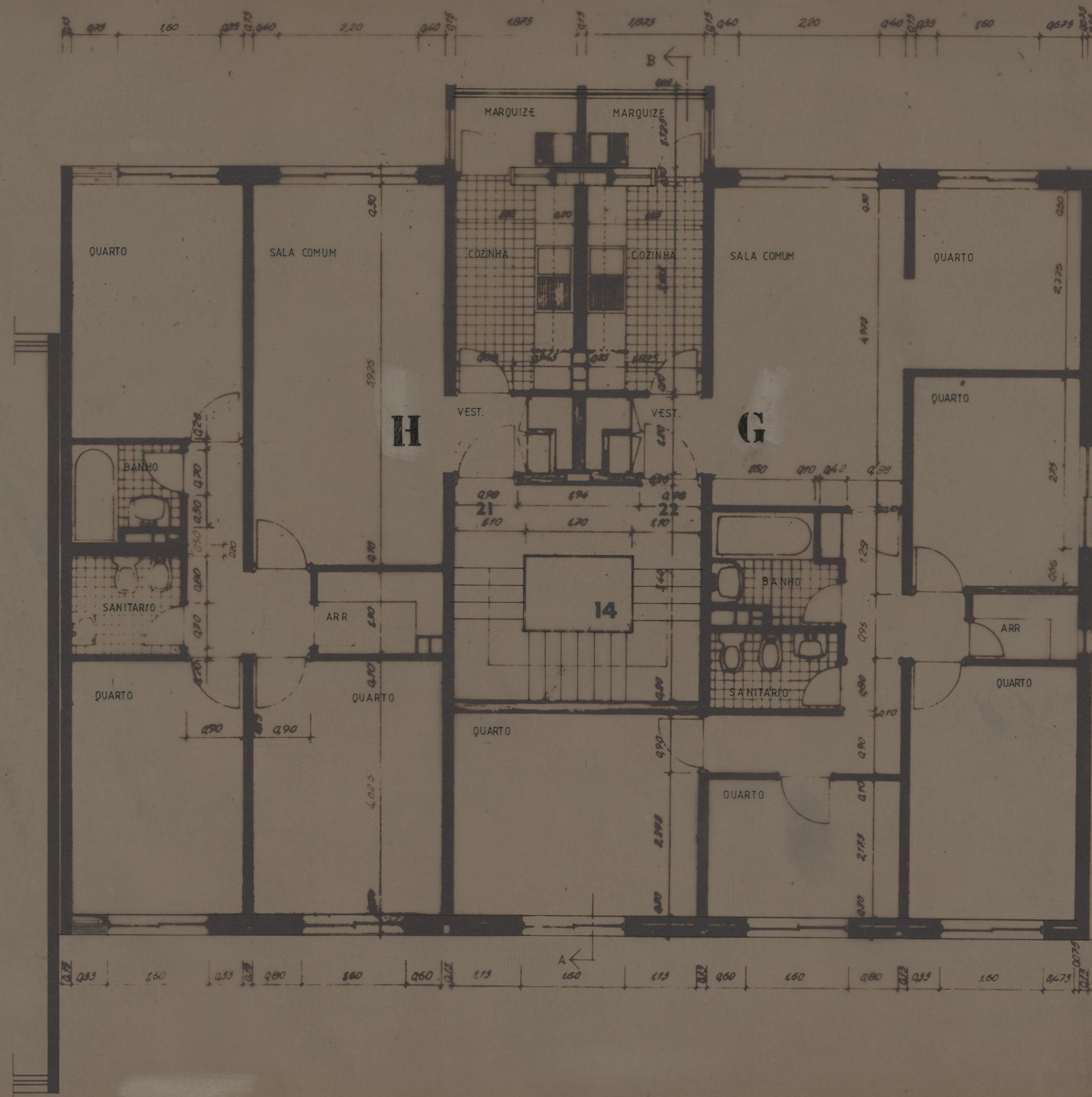
PLANTA DO 1º ANDAR (edificio 2)
