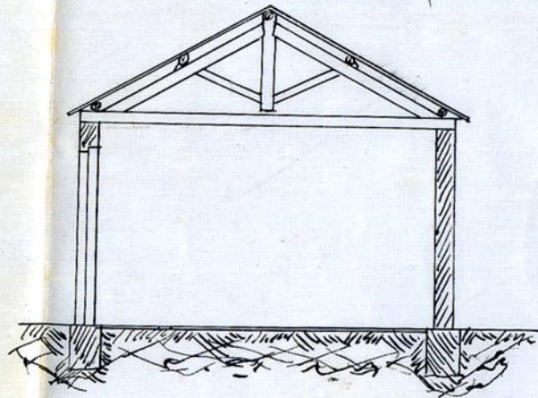
Corte transversal
