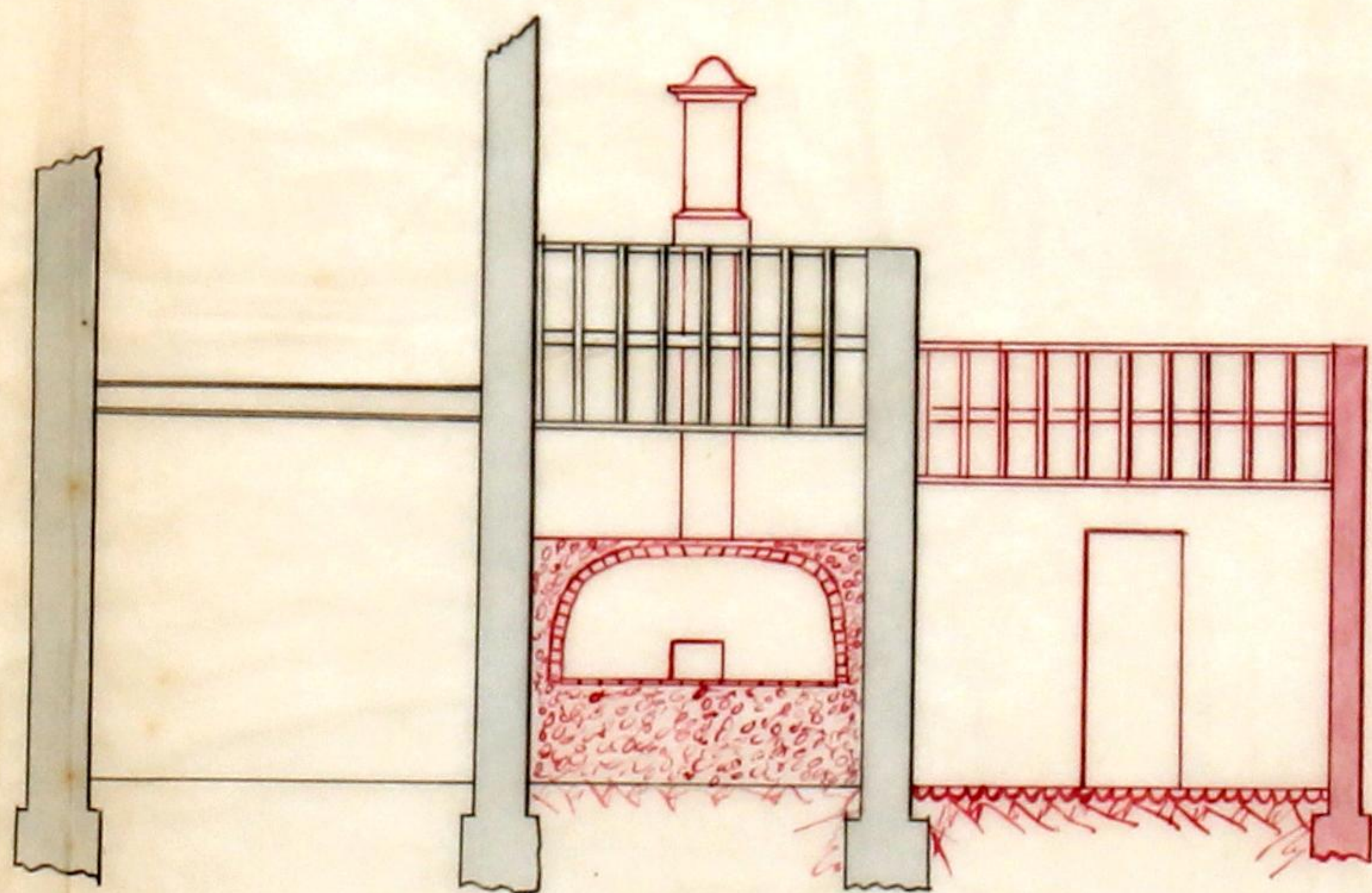
Corte por a linha a-b
