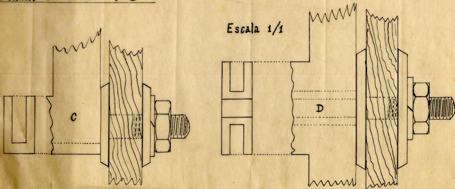
Detalhos dos Varões C e D
