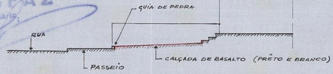
CORTE A
