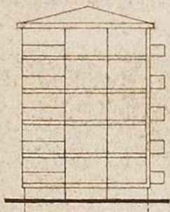
ALÇADO SUL
