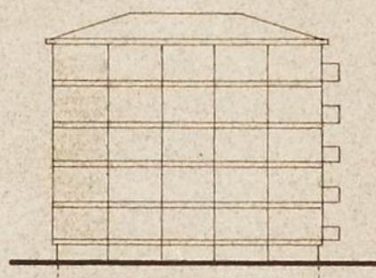
ALÇADO POENTE
