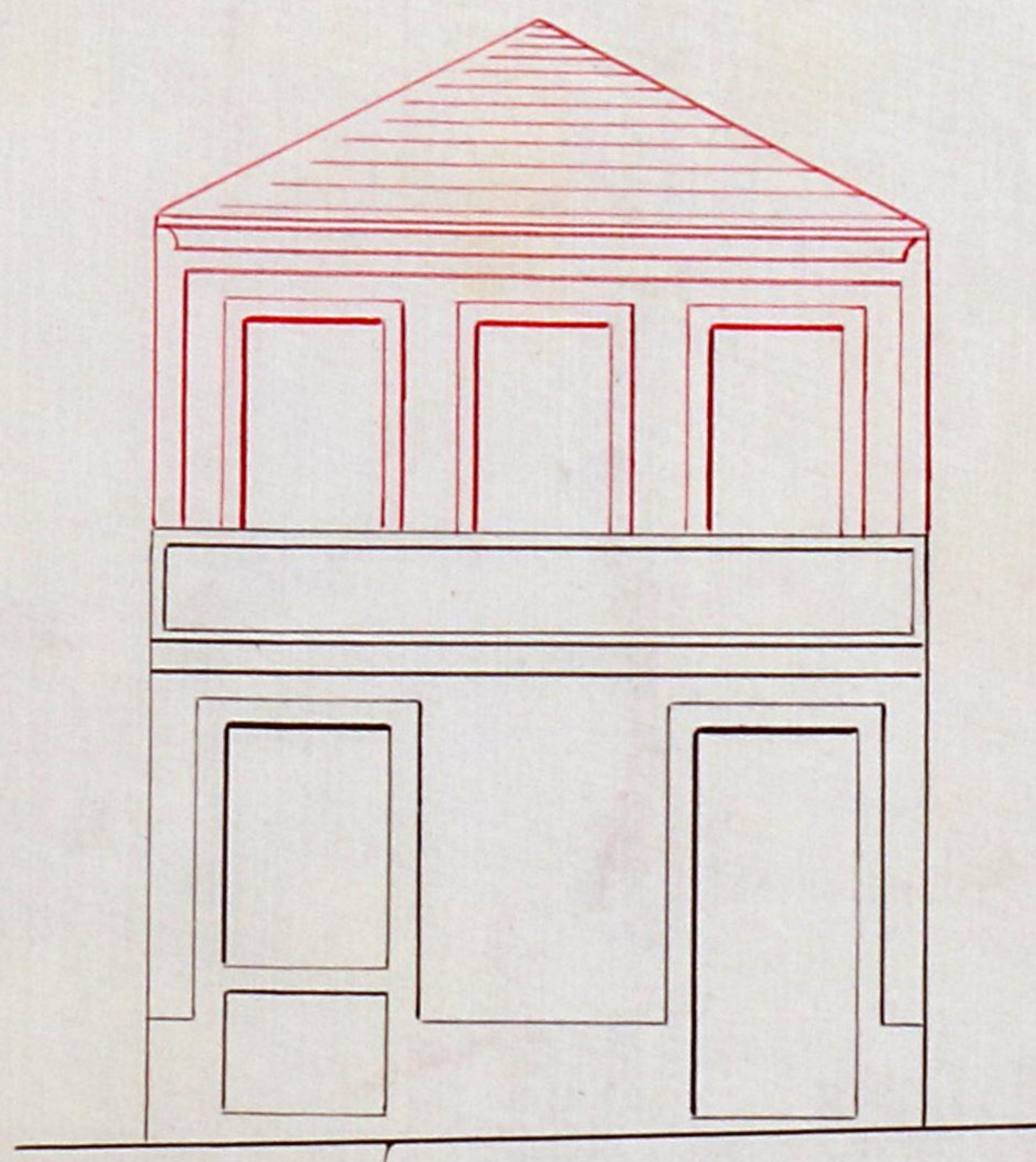
Alçado.
