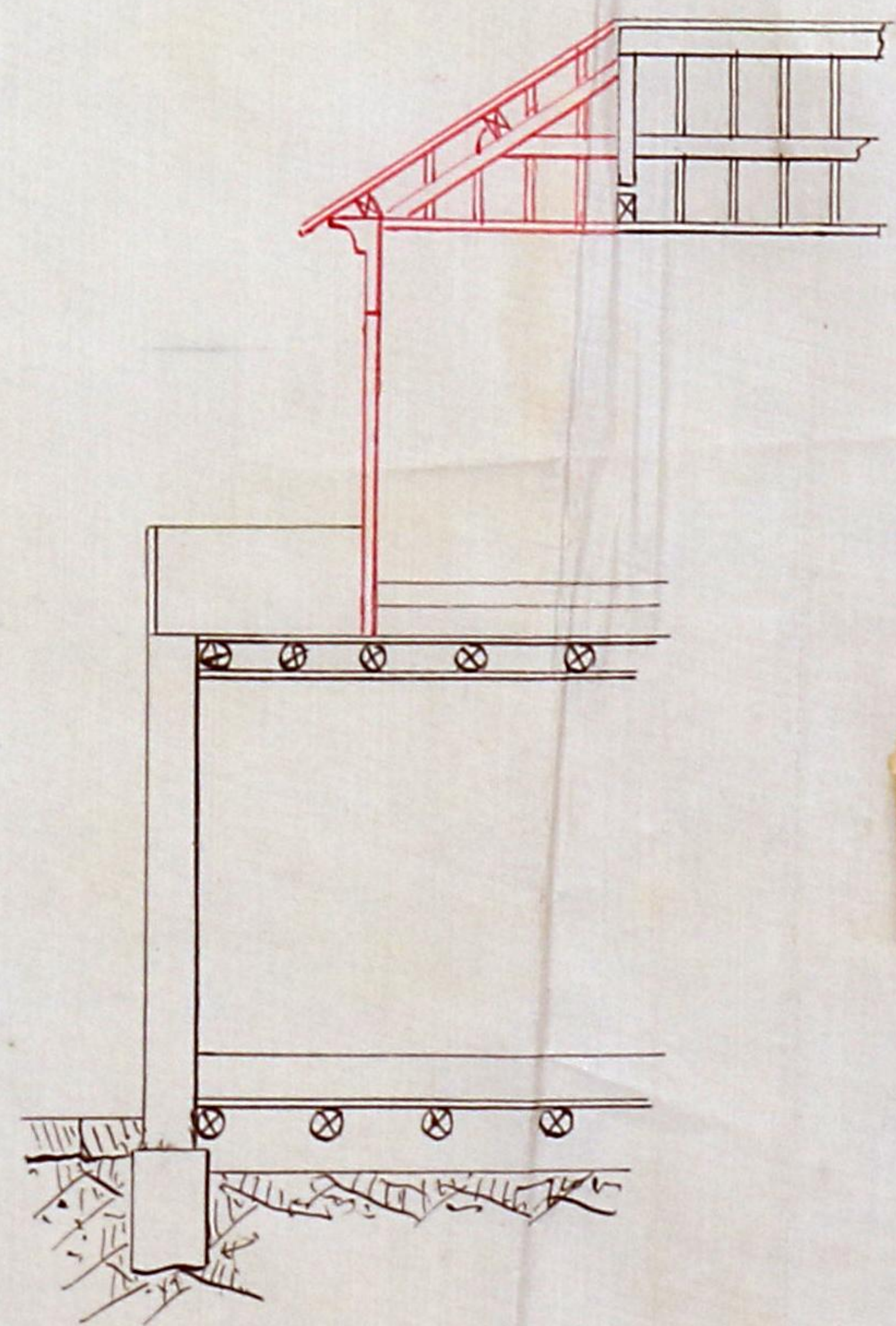
Corte vertical.
